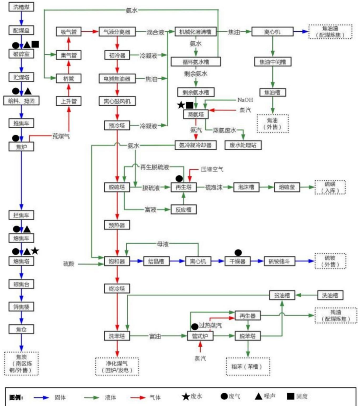
图4.3-1 工艺流程及产污环节图
